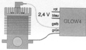
1-Zylinder-Motor
