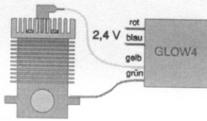
1-Zylinder-Motor
